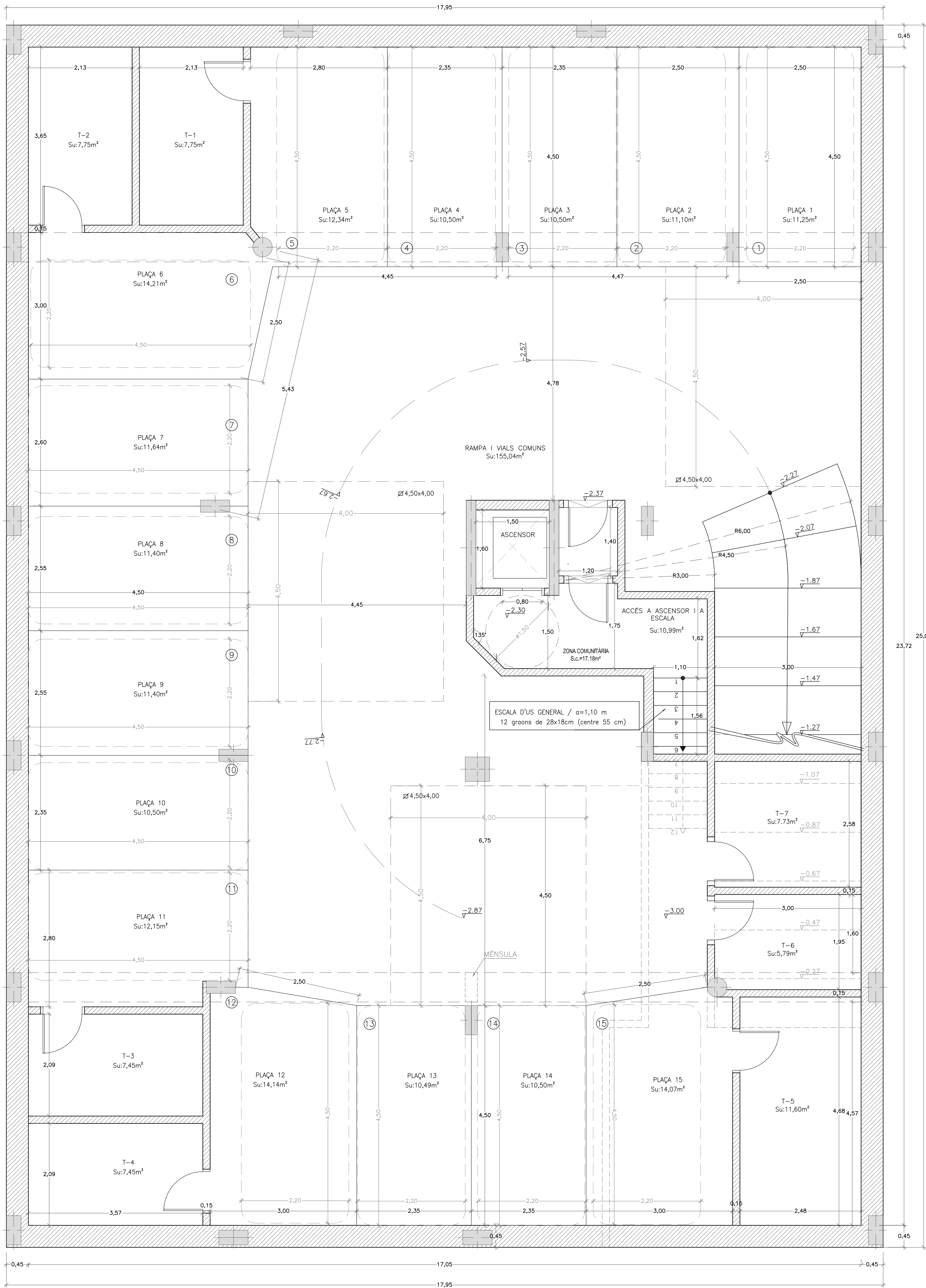
PLANTA SOTERRANI SUP.CONSTR.TOTAL=449,29m 2 escala 1/50
